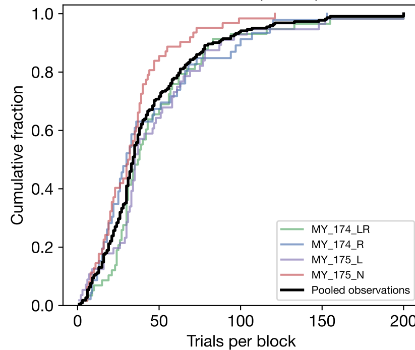
sub-01-04 (n=222)
