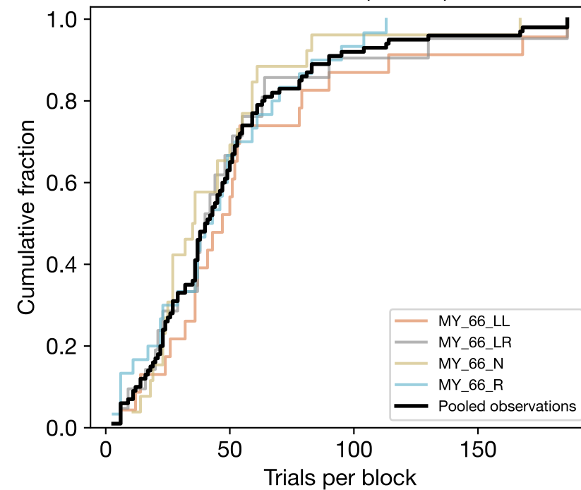
sub-05-08 (n=100)
